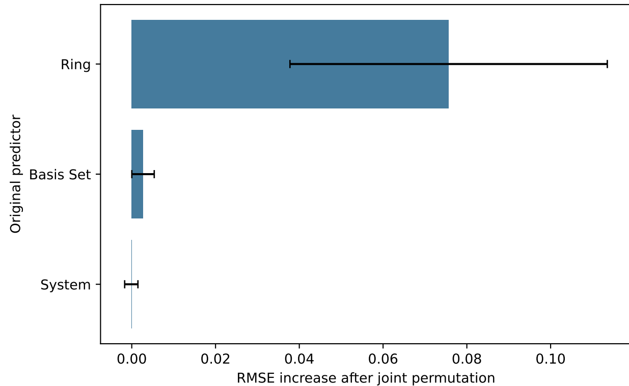
Grouped permutation importance: norm, |Q_2|(-1)
